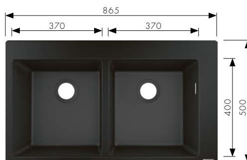
S510-F770 Встраиваемая мойка 370/370
