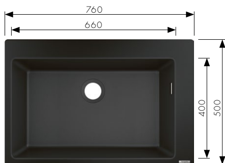
S510-F660 Встраиваемая мойка 660
