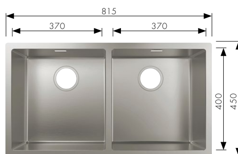
S719-U765 Мойка 370/370 для монтажа под столешницу Кухонный шкаф: 900 мм # 43430, -800 # 43922000 Система слива и перелива с ручным управлением
