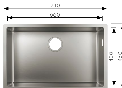
S719-U660 Мойка 660 для монтажа под столешницу Кухонный шкаф: 800 мм # 43428, -800 # 43921000 Система слива и перелива с ручным управлением
