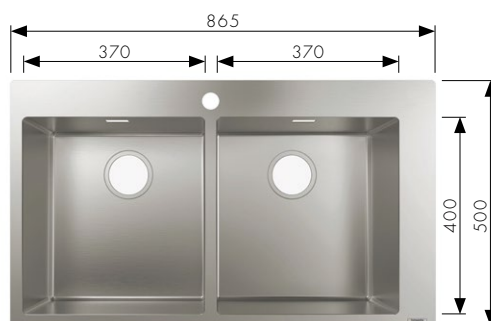
S711-F765 Встраиваемая мойка 370/370
