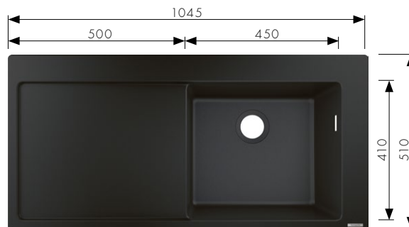
S514-F450 Встраиваемая мойка 450 с крылом
