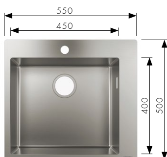
S711-F450 Встраиваемая мойка 450
