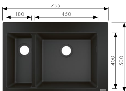
S510-F635 Встраиваемая мойка 180/450
